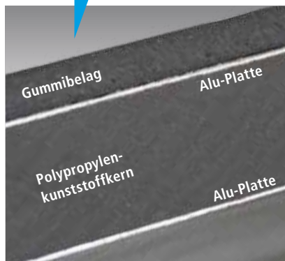
Unverrottbarer AluBiComp Boden
